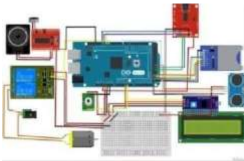
Gambar 2. Rangkaian Skematik Keseluruhan Sistem
