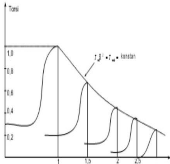
Gambar 4. Karakteristik Torsi kecepatan untuk kendali frekuensi
