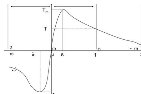
Gambar 2. Karakteristik Torsi terhadap kecepatan
