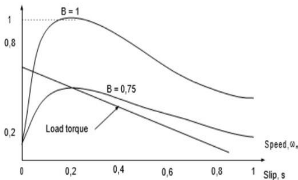
Gambar 3. Karakteristik torsi terhadap kecepatan dengan harga tegangan yang bervariasi
