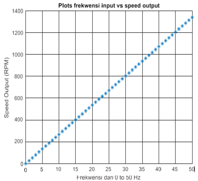
Gambar 6. Grafik Frekwensi dan Kecepatan
